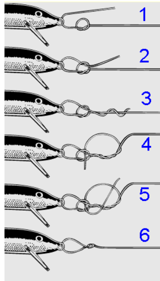
Nœud de Rapala
